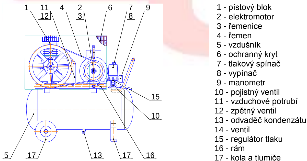
Obr. 5 - Celkový pohled na kompresor C-50.AB515
