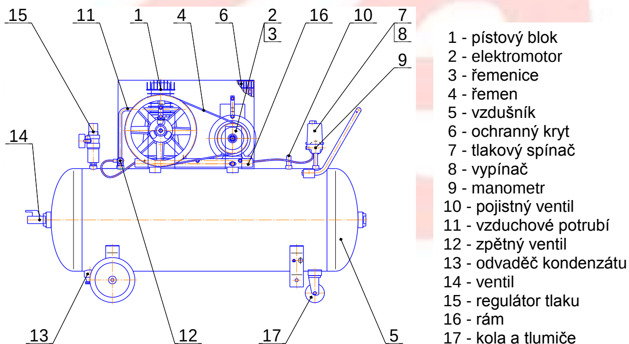
Obr. 7 - Celkový pohled na kompresor C-200.AB515
