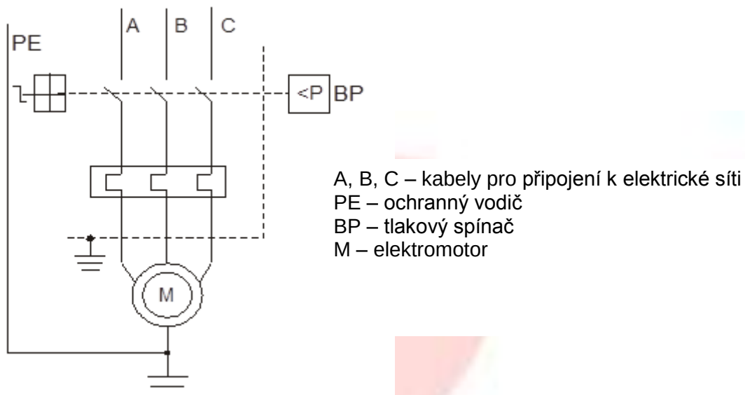
Obrázek A.1 – Schéma elektrických obvodů
