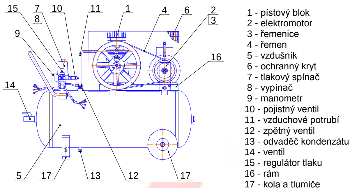
Obr. 6 - Celkový pohled na kompresor C-100.AB515
